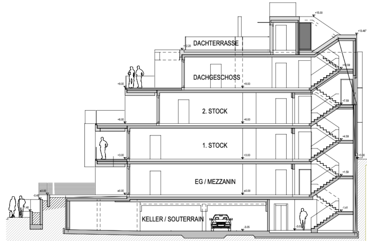
SCHNITT DURCH STIEGENHAUS
